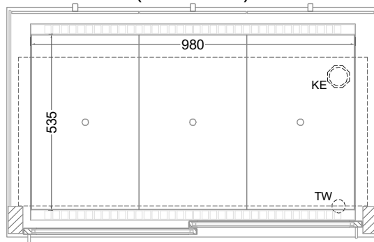
(Grundriss)
