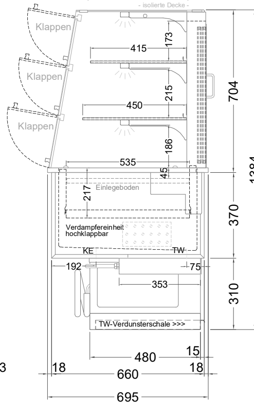
(Seitenansicht)
