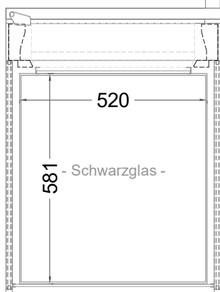
(Grundriss)
