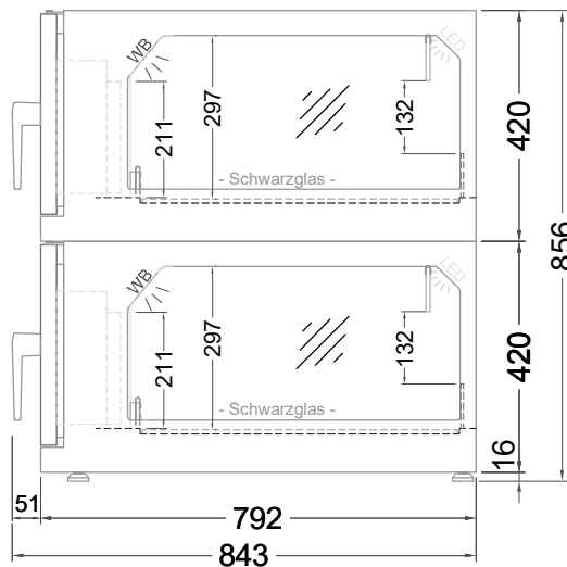
(Seitenansicht)
