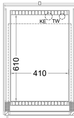
(Grundriss)
