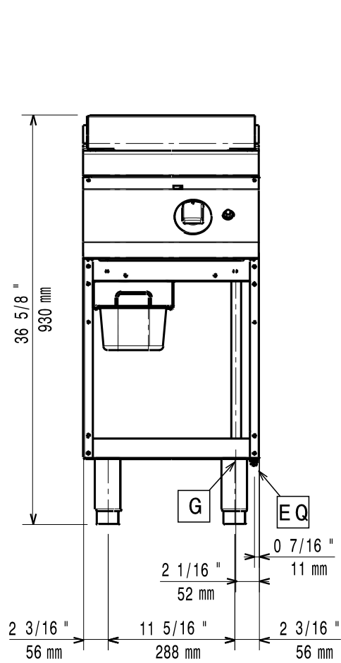
[Vorderansicht]
