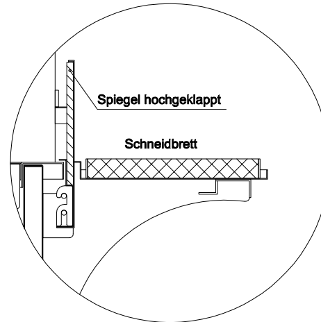
(Detail Spiegelsystem)
