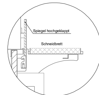
(Detail Spiegelsystem)
