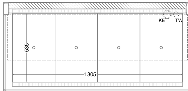
(Grundriss)
