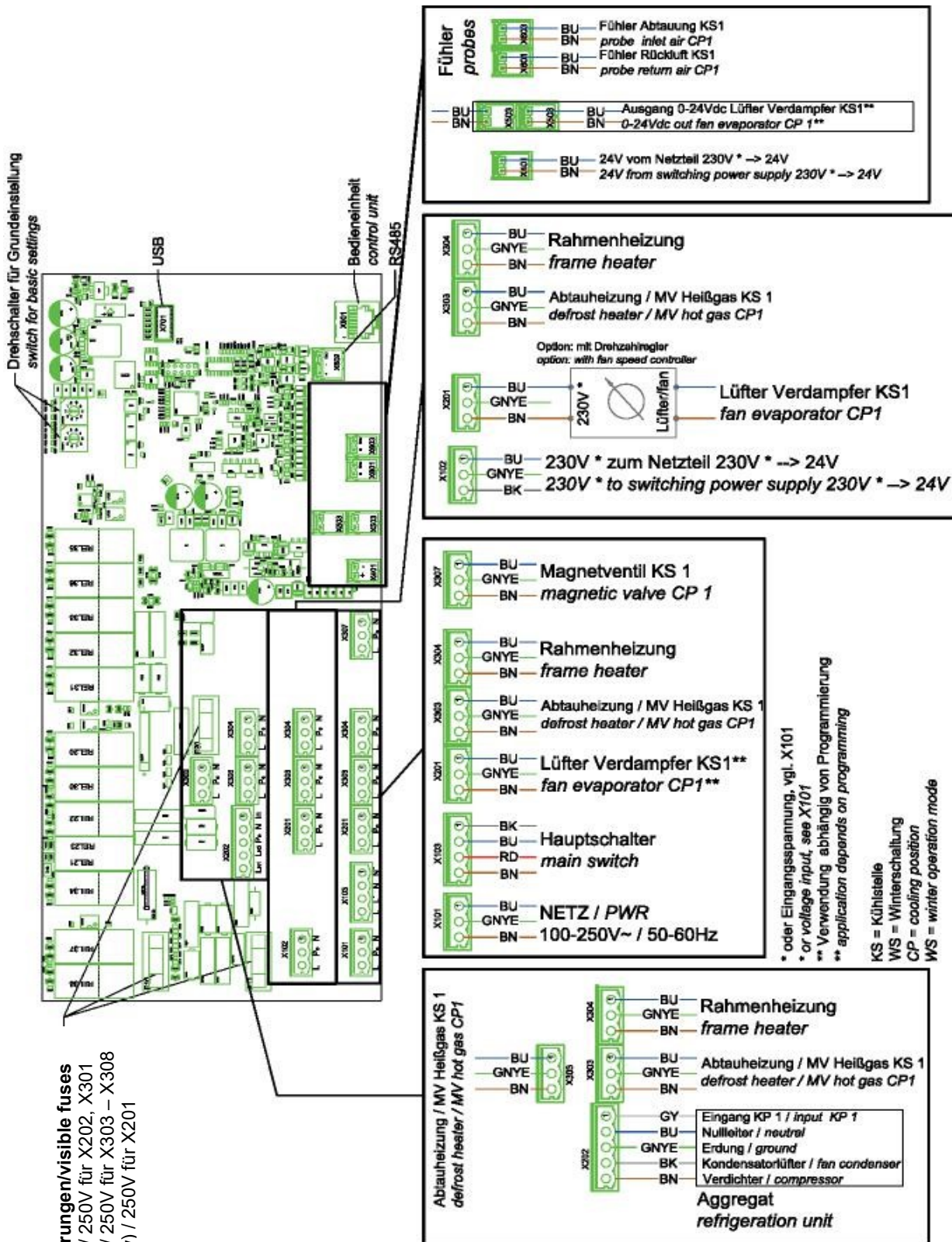
Abbildung 5: Platine Übersicht
