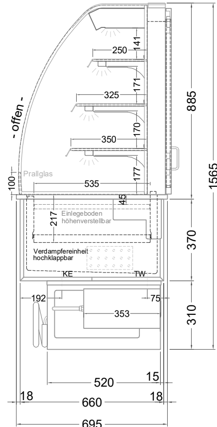
(Seitenansicht)
