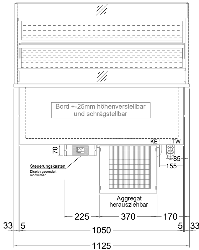
(Grundriss)
