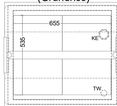
(Grundriss)
