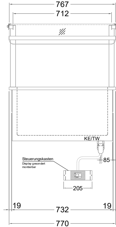
(Bedienseite)
