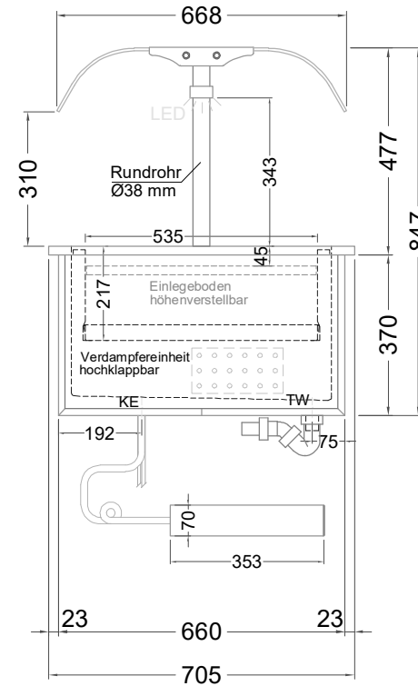
(Seitenansicht)
