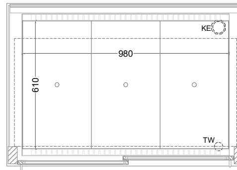
(Grundriss)
