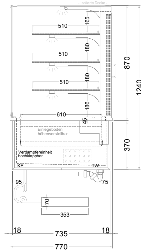
(Seitenansicht)
