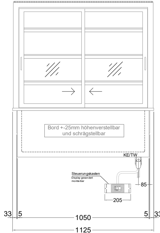
(Bedienseite)
