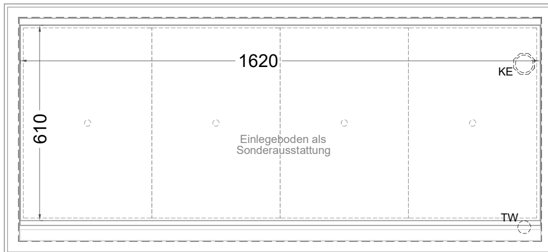
(Grundriss)
