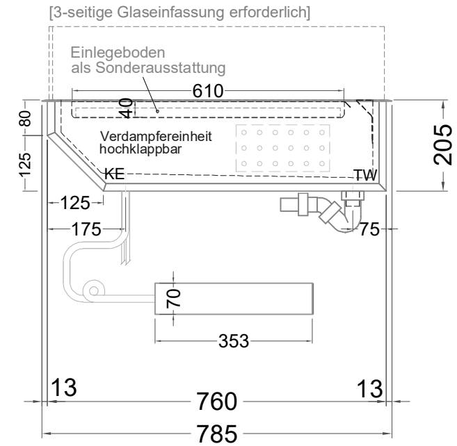
(Seitenansicht)
