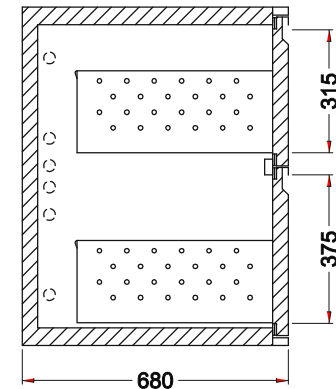
Schnitt L1
