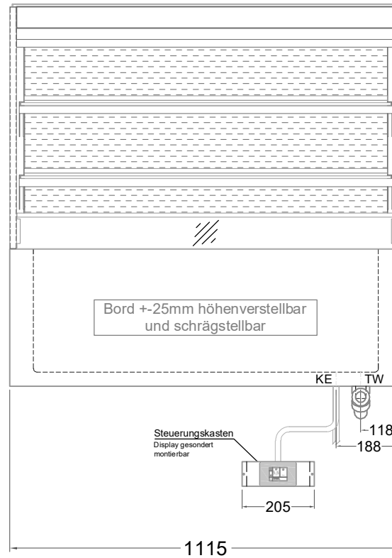
(Vorderseite)
