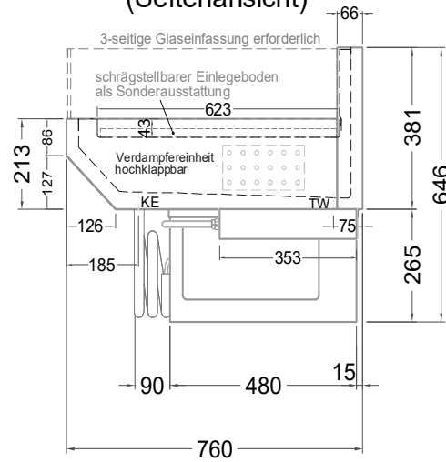
(Seitenansicht)
