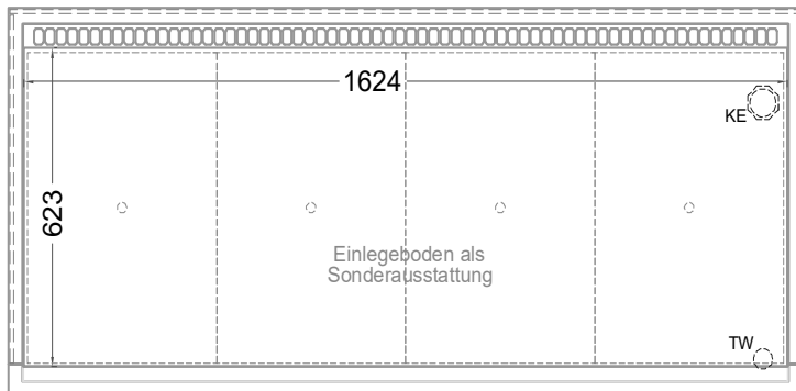
(Grundriss)
