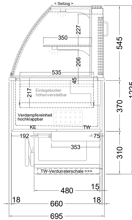
(Seitenansicht)
