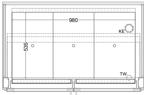
(Grundriss)
