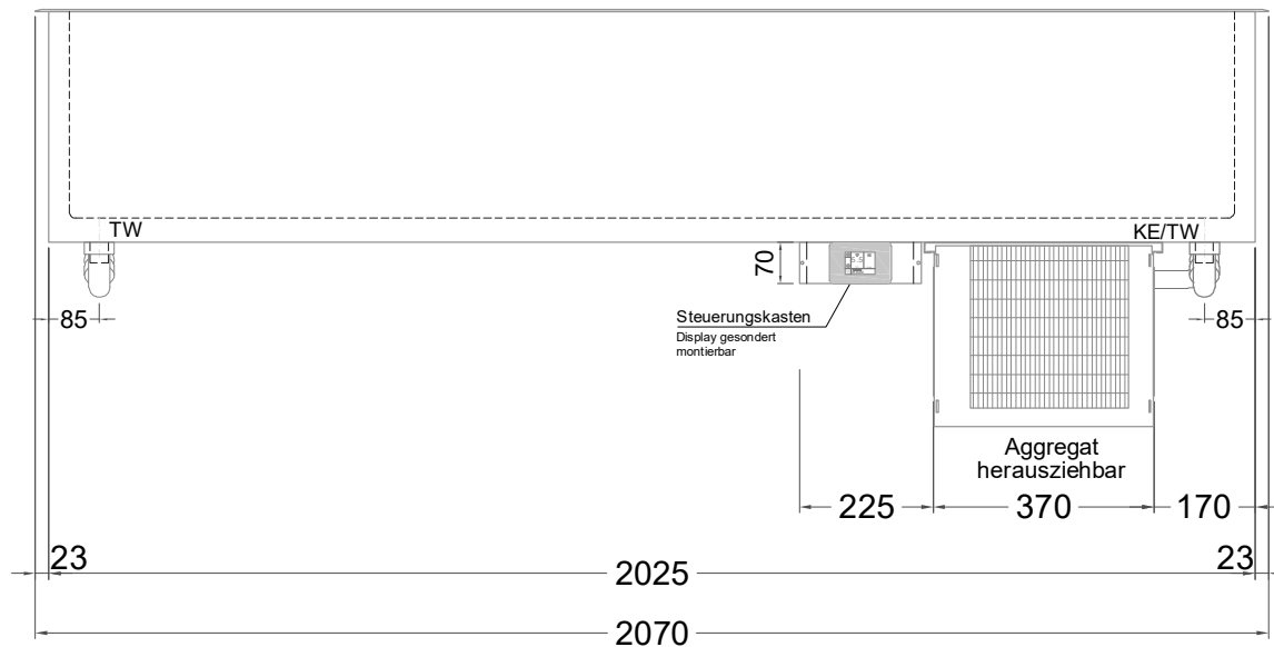
(Grundriss)
