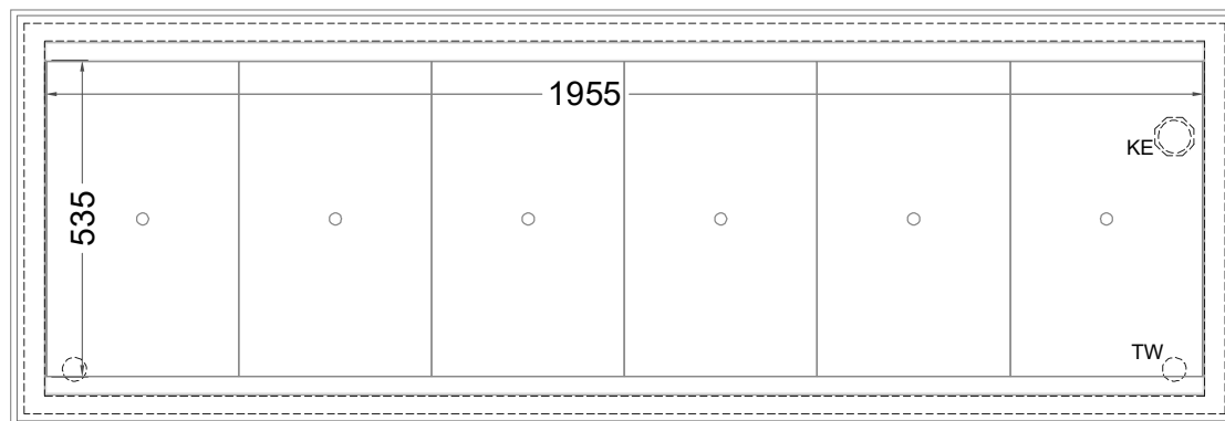
(Grundriss)
