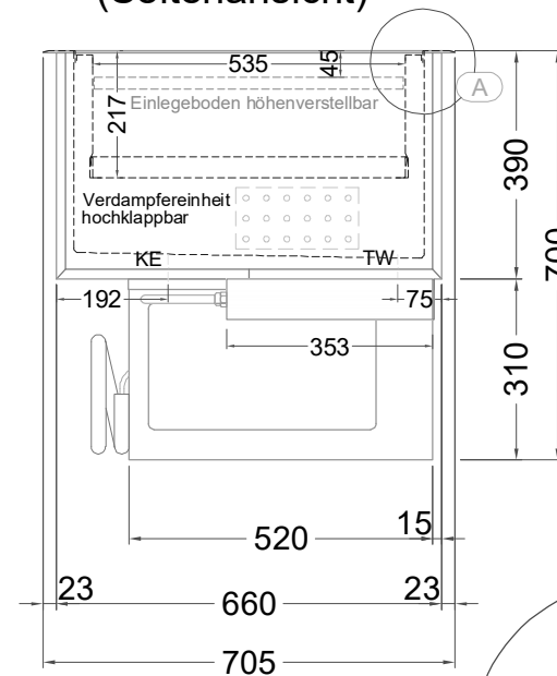
(Seitenansicht)
