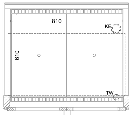
(Grundriss)
