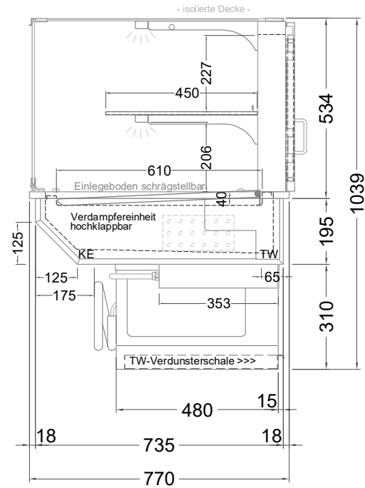
(Seitenansicht)
