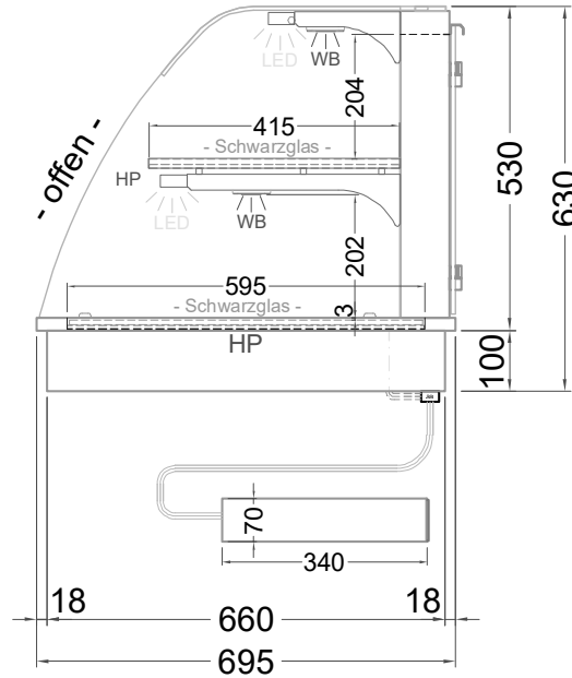
(Seitenansicht)
