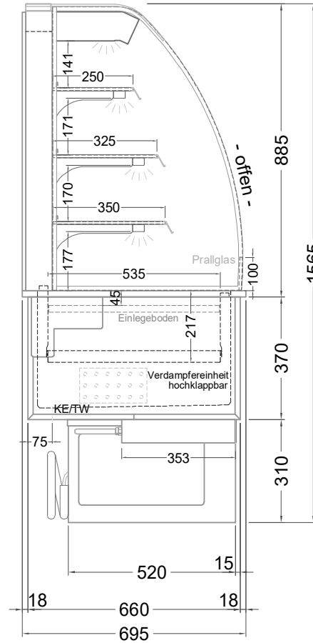
(Seitenansicht)
