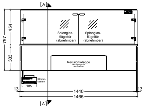
(Bedienseite)
