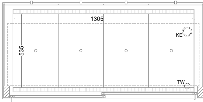
(Grundriss)
