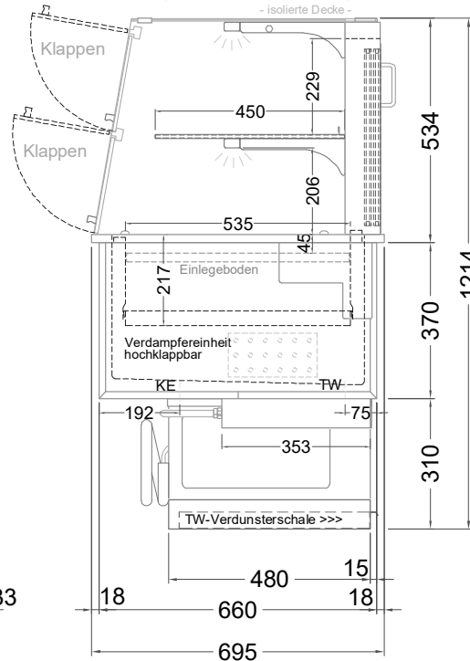
(Seitenansicht)
