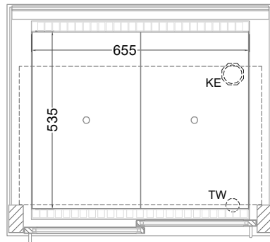
(Grundriss)
