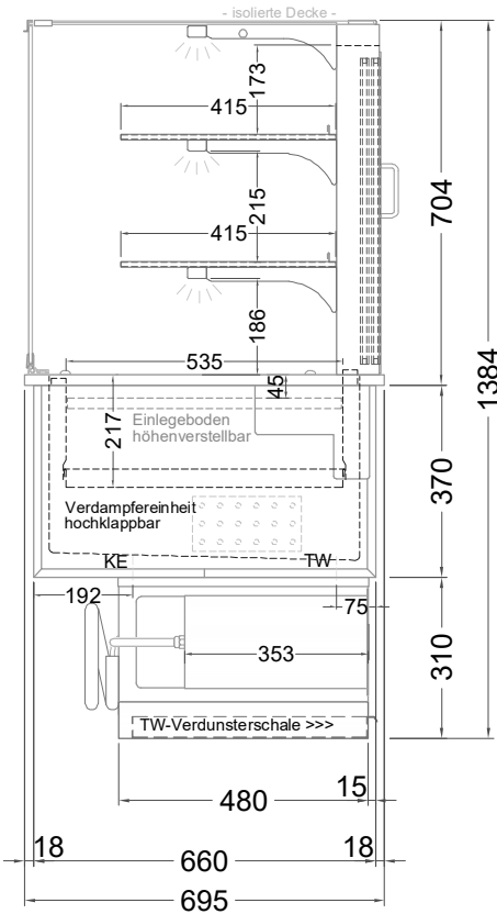
(Seitenansicht)
