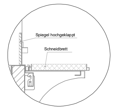
(Detail Spiegelsystem)
