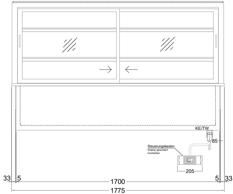
(Bedienseite)
