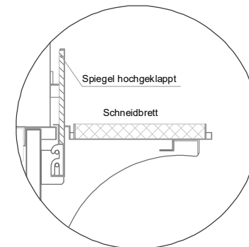
(Detail Spiegelsystem)
