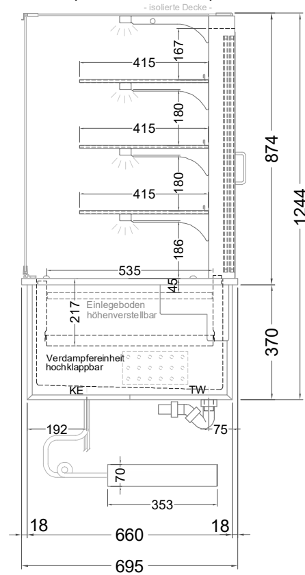
(Seitenansicht)
