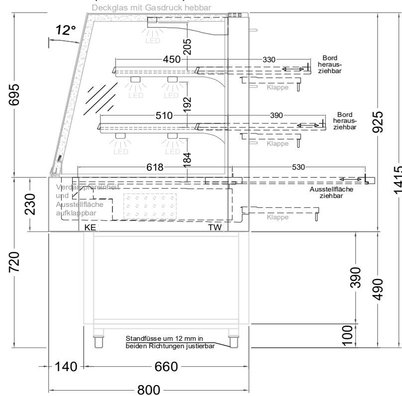
(Seitenansicht)
