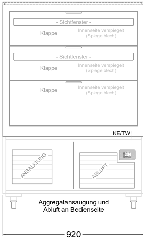
(Bedienseite)
