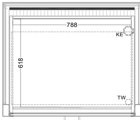
(Grundriss)
