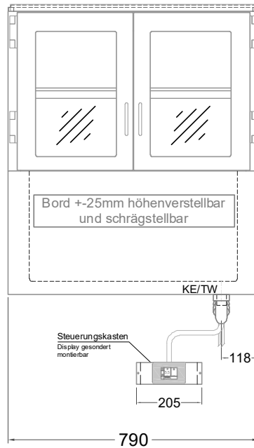
(Bedienseite)
