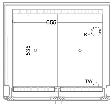
(Grundriss)
