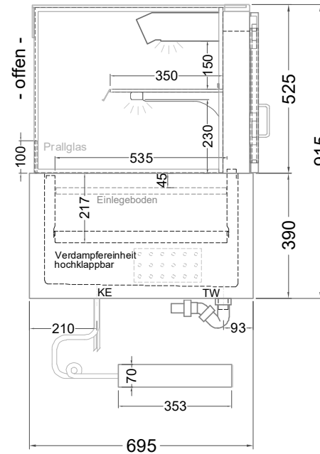
(Seitenansicht)
