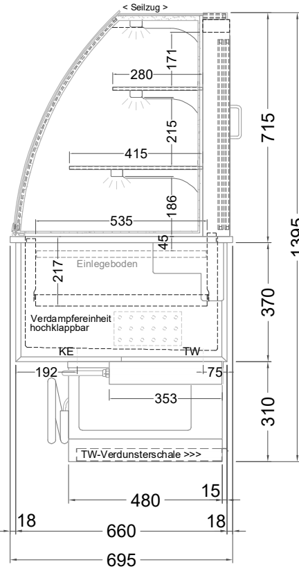
(Seitenansicht)
