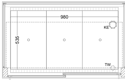
(Grundriss)
