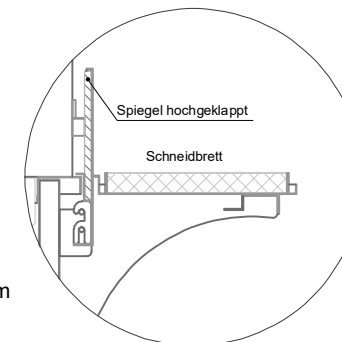
(Detail Spiegelsystem)
