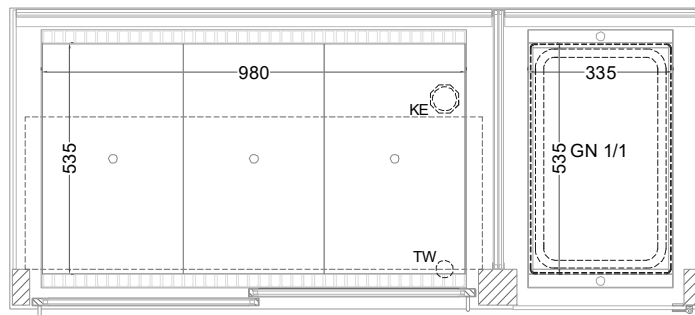
(Grundriss)
