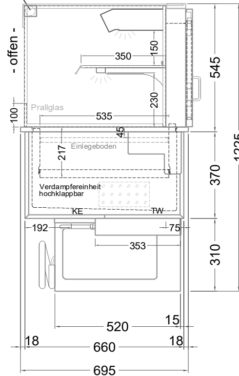
Rollo (Seitenansicht)
