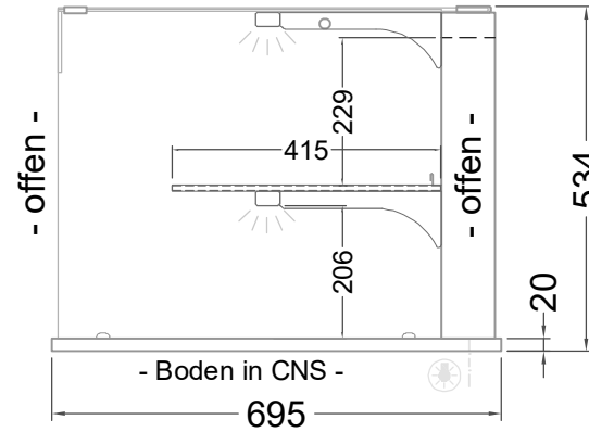
(Seitenansicht)
