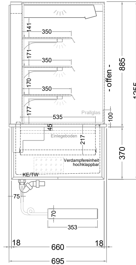
(Seitenansicht)
