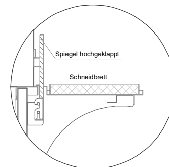
(Detail Spiegelsystem)
