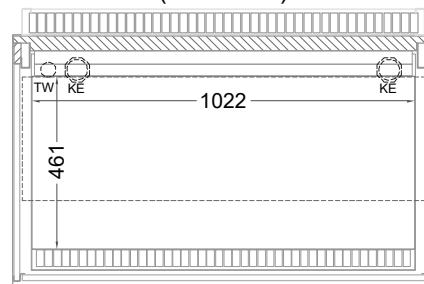
(Grundriss)
