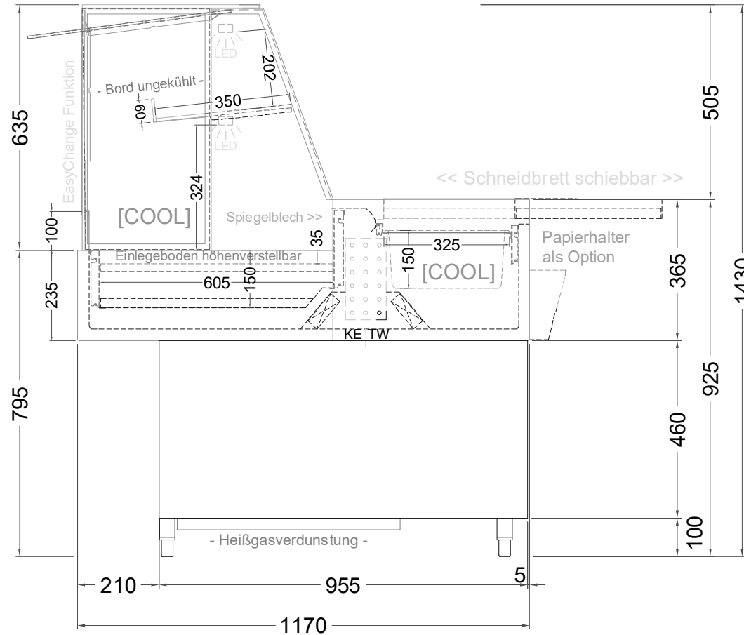
(Seitenansicht)
