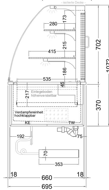
(Seitenansicht)
