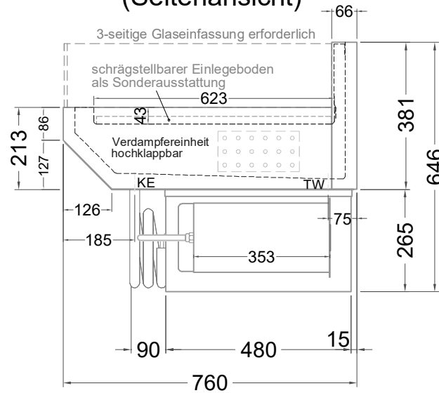
(Seitenansicht)
