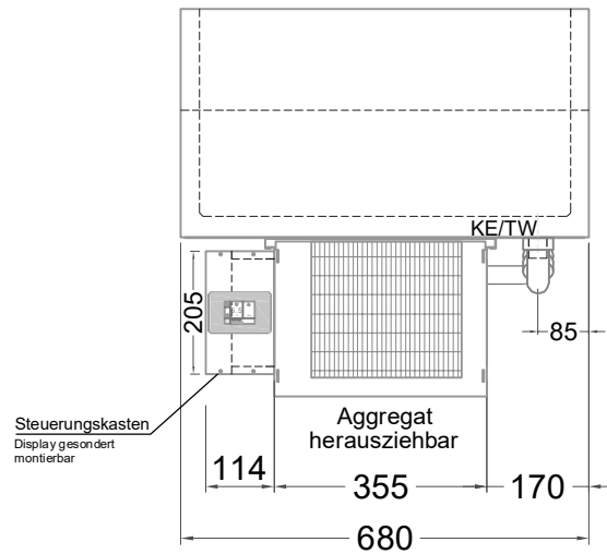
(Grundriss)
