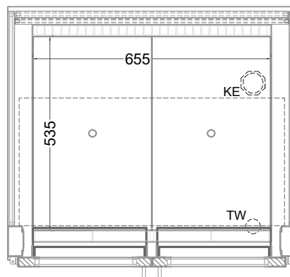
(Grundriss)
