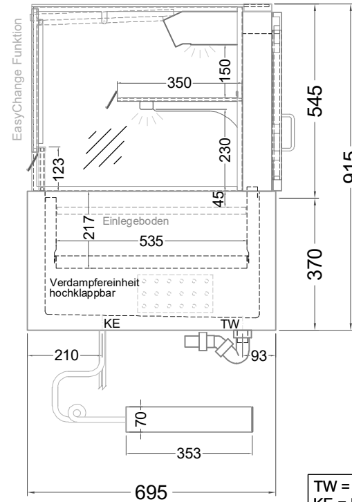
(Seitenansicht)
