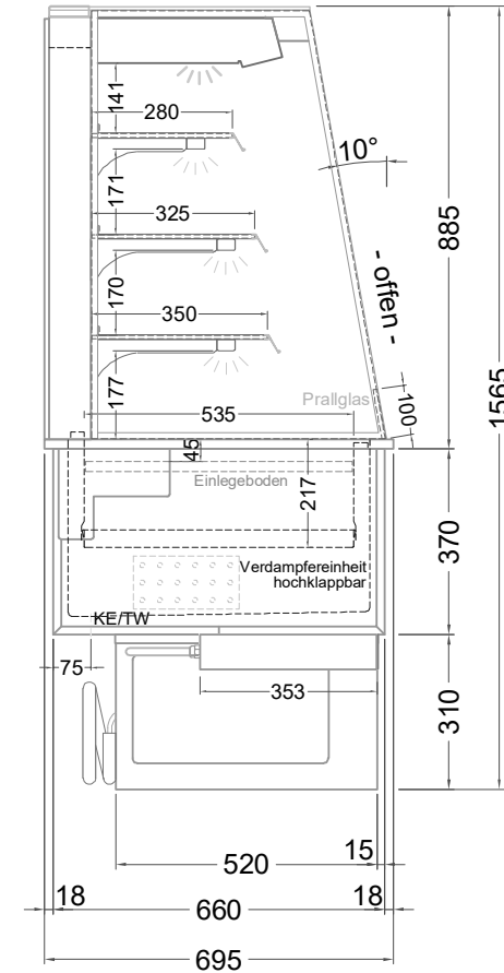
(Seitenansicht)
