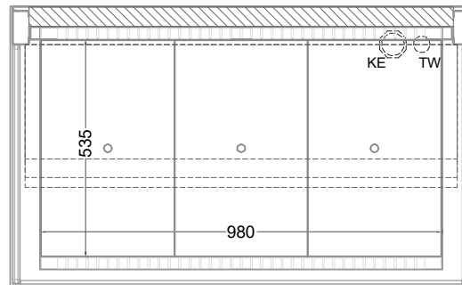
(Grundriss)
