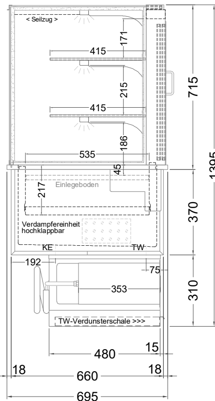
(Seitenansicht)
