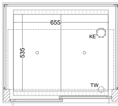
(Grundriss)
