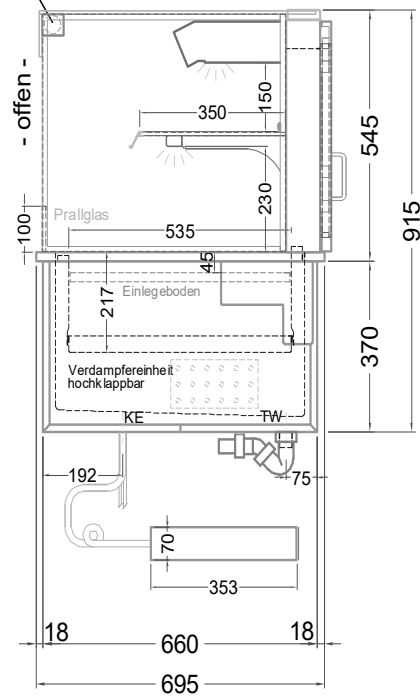
Rollo (Seitenansicht)
