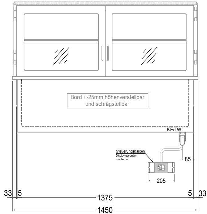
(Bedienseite)
