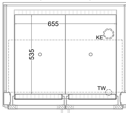
(Grundriss)
