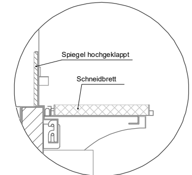
(Detail Spiegelsystem)
