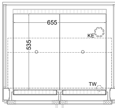
(Grundriss)
