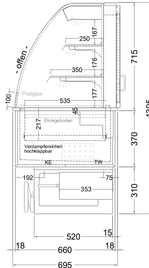
(Seitenansicht)
