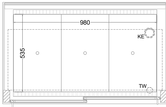
(Grundriss)
