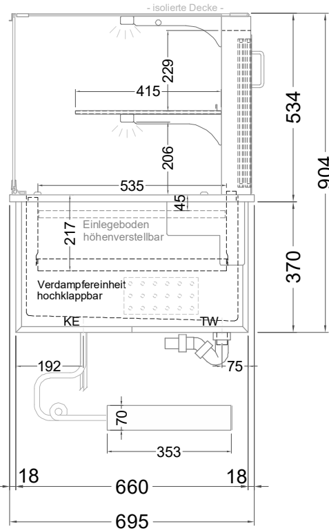
(Seitenansicht)
